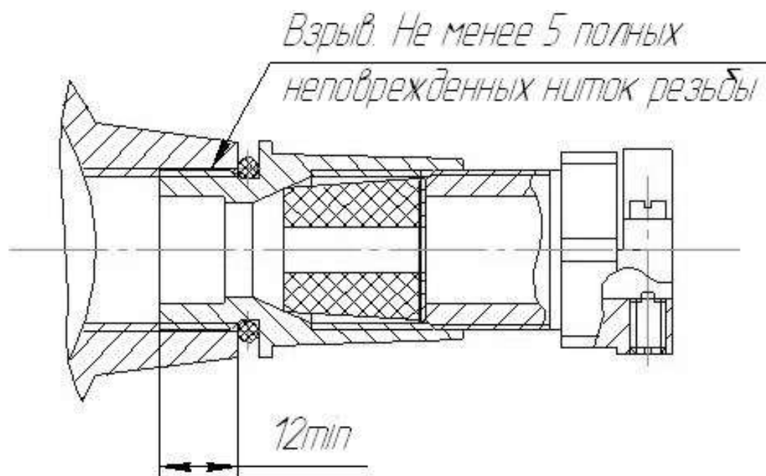
Рис. 2А Чертеж средств взрывозащиты ввода бронированного кабеля с зажимом для металлорукава (маркировка взрывозащиты 1Ex db IIC T6 Gb X)
