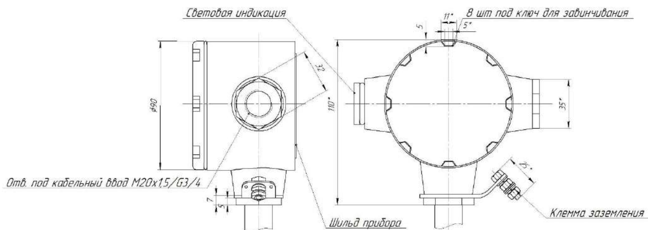
Рис.2 Корпус из алюминиевого сплава (IP65/IP67).
